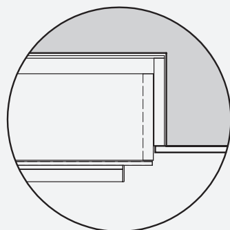
Einbau UP mit Einbaurahmen Encastré avec cadre à encastrer
